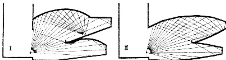
نمودار ۱/۳/۱/۵/۱، ۱. سقف شکسته که بازتاب‌های یکنواخت به‌وجود می‌آورد.
